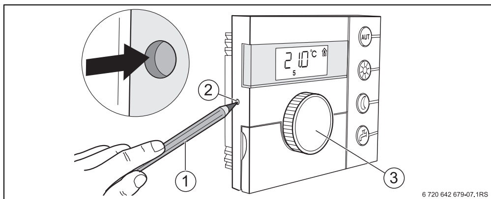
Рис. 7 Потайная кнопка
