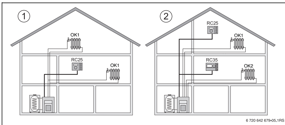
Рис. 2 Варианты управления отопительной установкой с одним или двумя отопительными контурами
